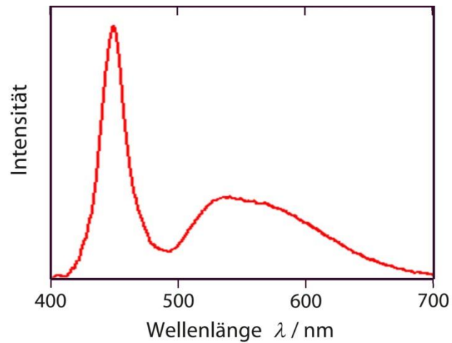
Notebookbildschirm/weiße LED
