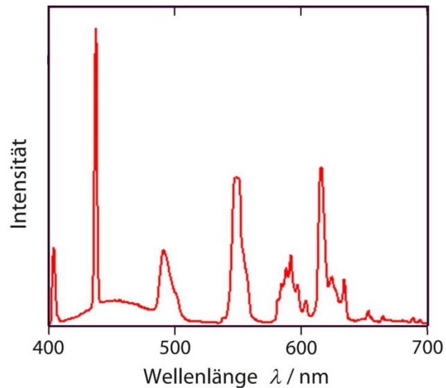
Energiesparlampe/Leuchtstoffröhre
