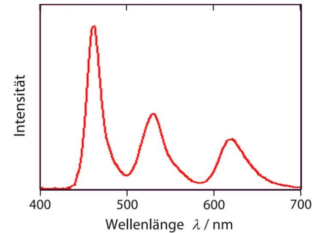
OLED-Smartphone Bildschirm
